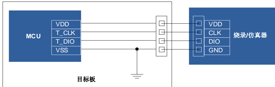
ICP 模式 Flash Writer 编程连接示意图
