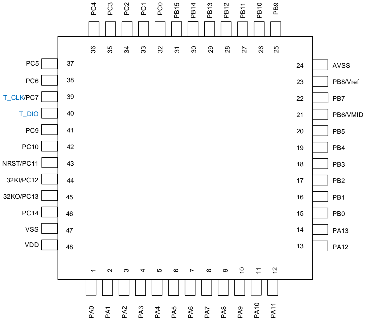
48PIN 管脚配置图 适用于 LQFP48、QFN48 封装
